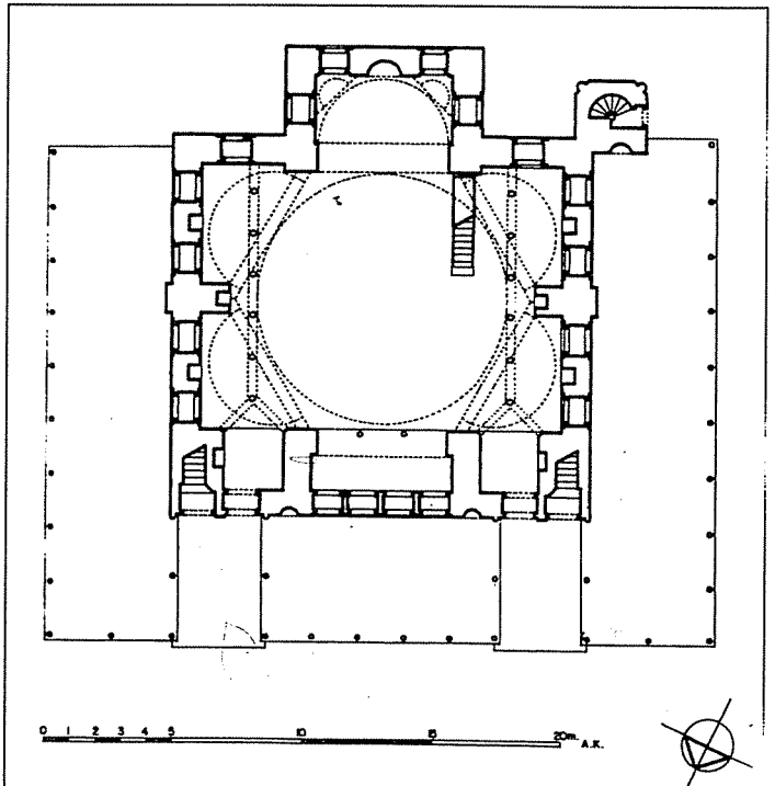
İvaz Efendi Camii'nin planı. Kuran, Mimar Sinan
