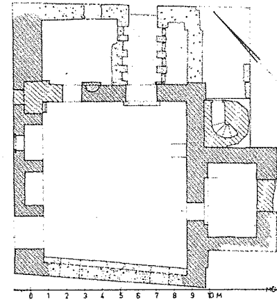
Kasım Ağa Mescidi planı
