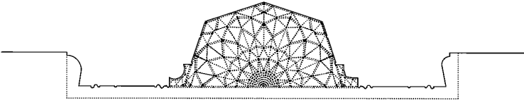
8 b - Plân
