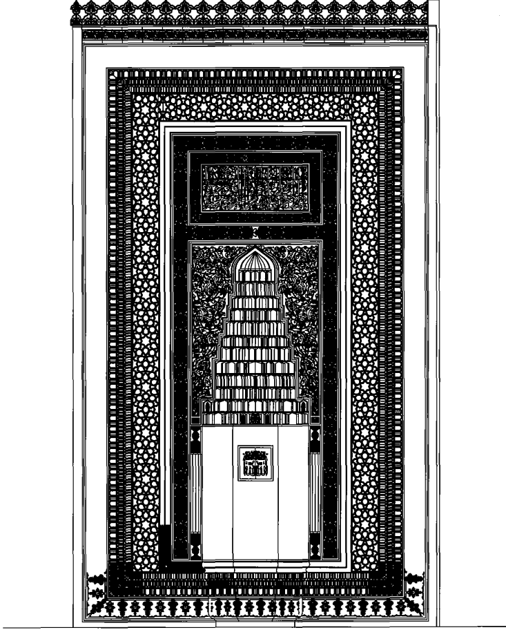
7 a - Görünüş
